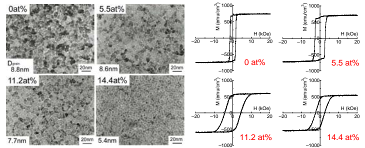
CoPtCr-SiO 2 媒体のSiO 2 組成に対するTEM像とヒステリシスループ
