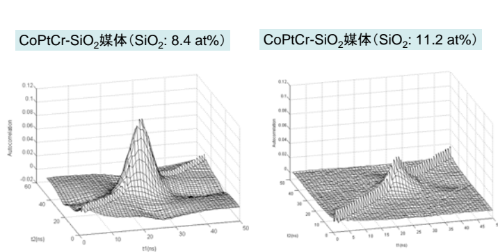
自己相関を用いた磁気記録再生波形ノイズ成分解析
