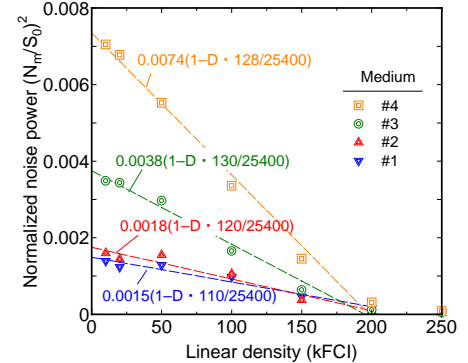
逆磁区ノイズの記録密度依存性
