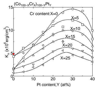
K_u のPt組成依存性
