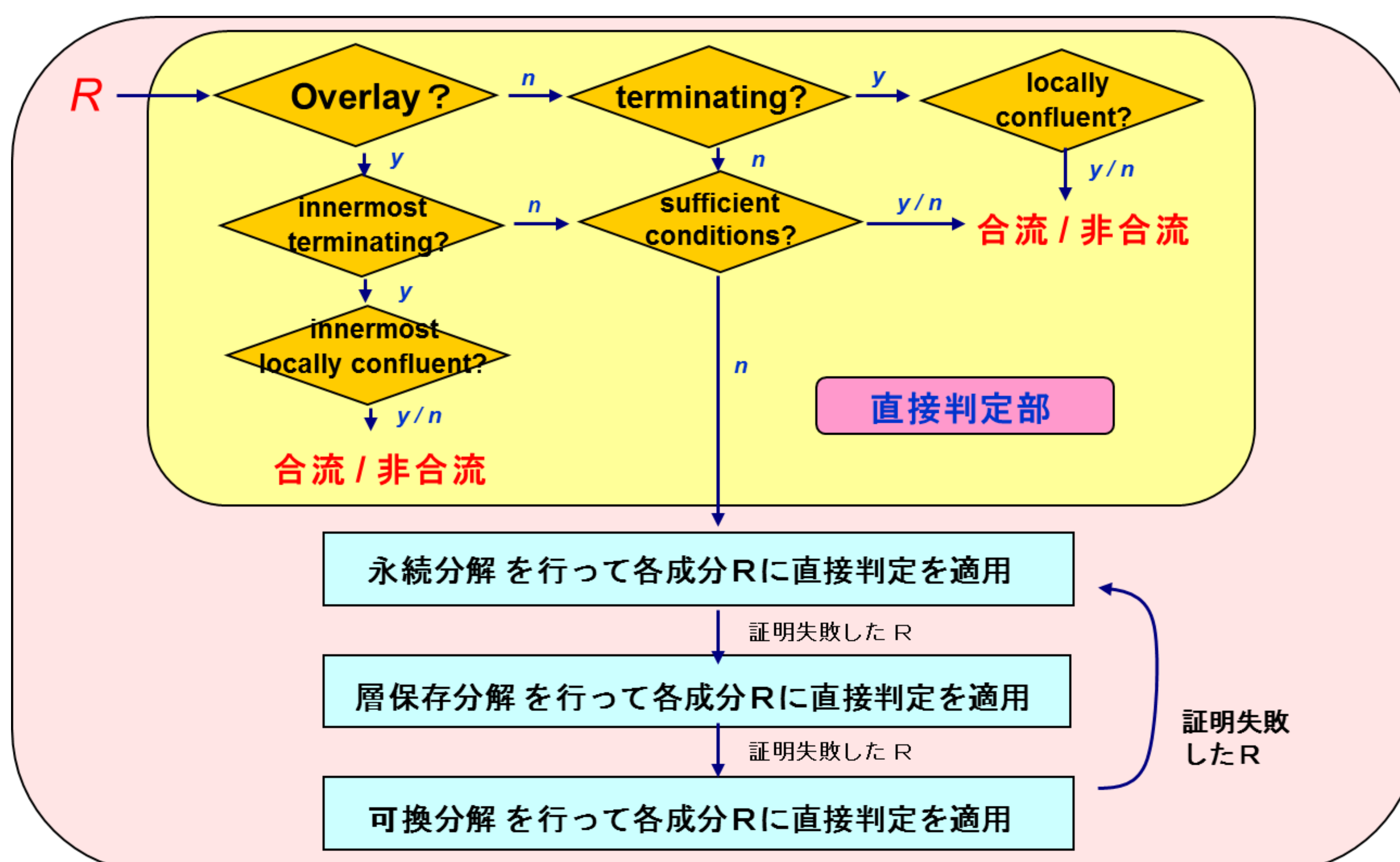
合流性自動判定システムACPの概要
