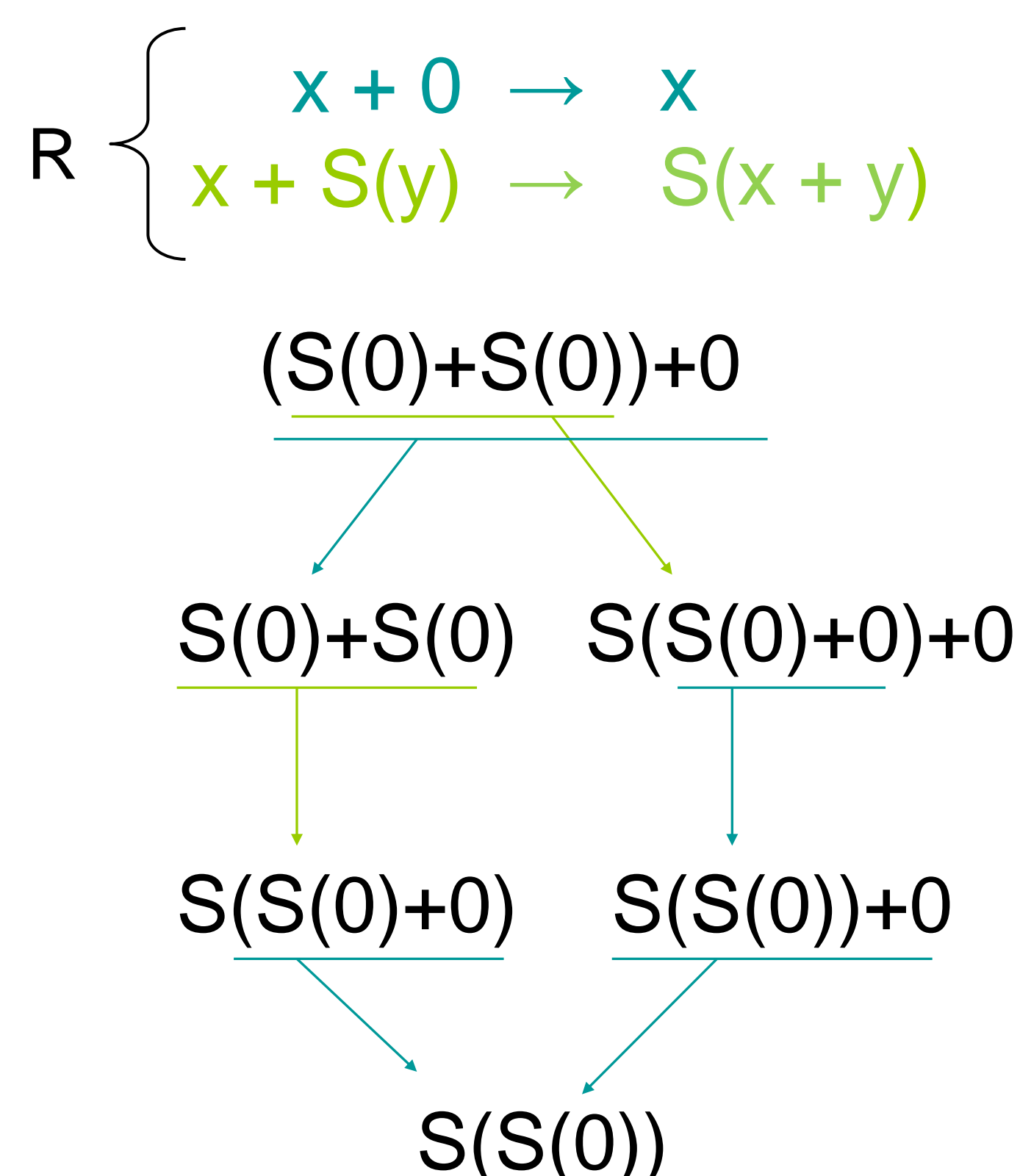
書き換えシステムの合流性
