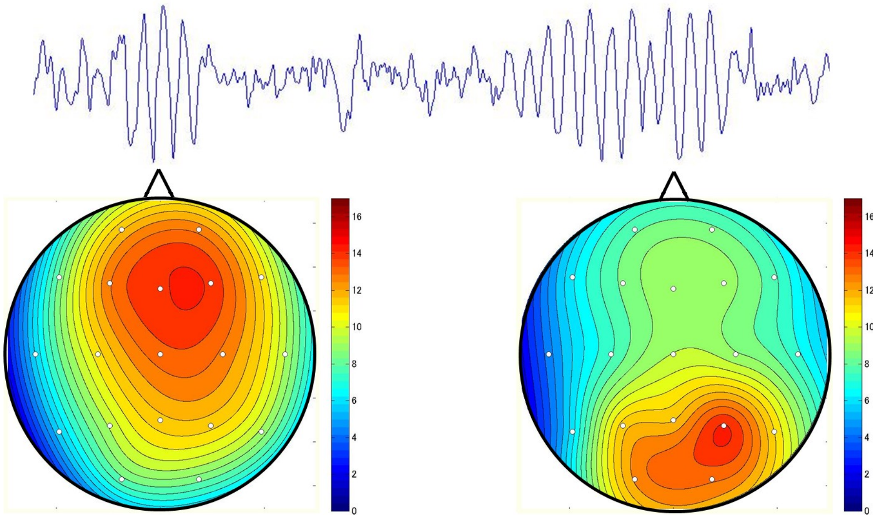
眠気に伴って出現するα波(上段)、おおよび眠気が中程度の時(下段左)と強い時(下段右)のα波のトポグラフ
