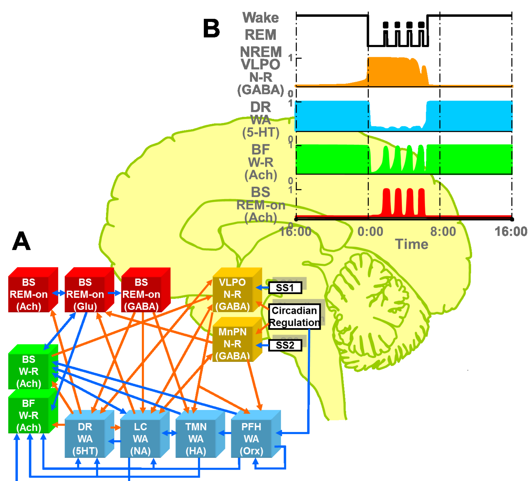
(A) ヒトの睡眠・覚醒状態の遷移を制御する神経系の解剖学・生理学的知見に基づく神経回路モデル。(B) ヒトの睡眠・覚醒リズムのシミュレーション結果。
