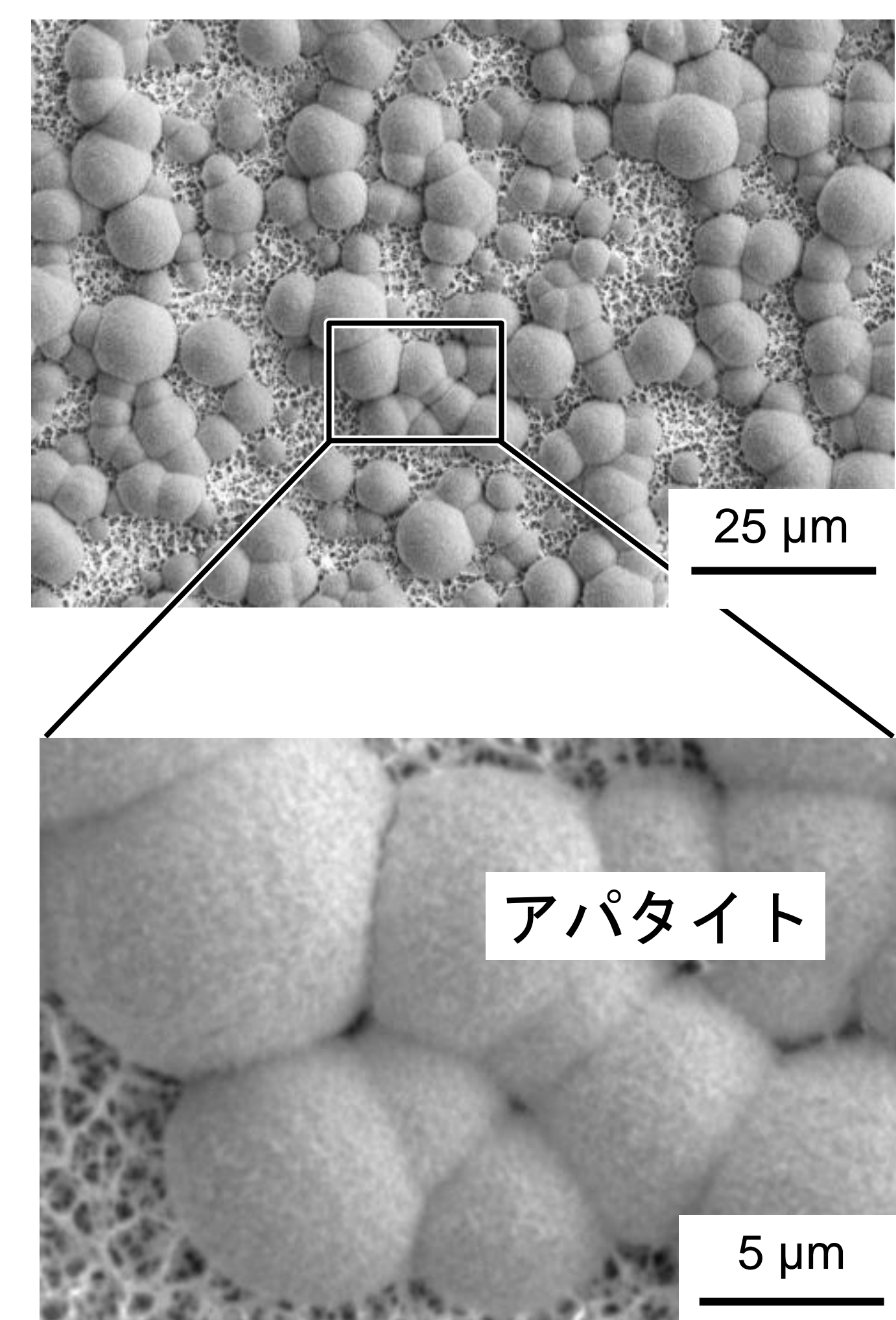
図6 \text{NaOH-NH}_4\text{OH} -加熱処理後、SBFに7日間浸漬したチタン金属のSEM写真
