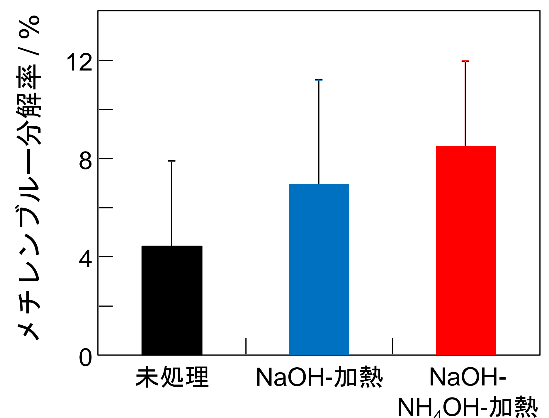
図7 種々の条件で表面処理したチタン金属の可視光下におけるメチレンブルー分解率
