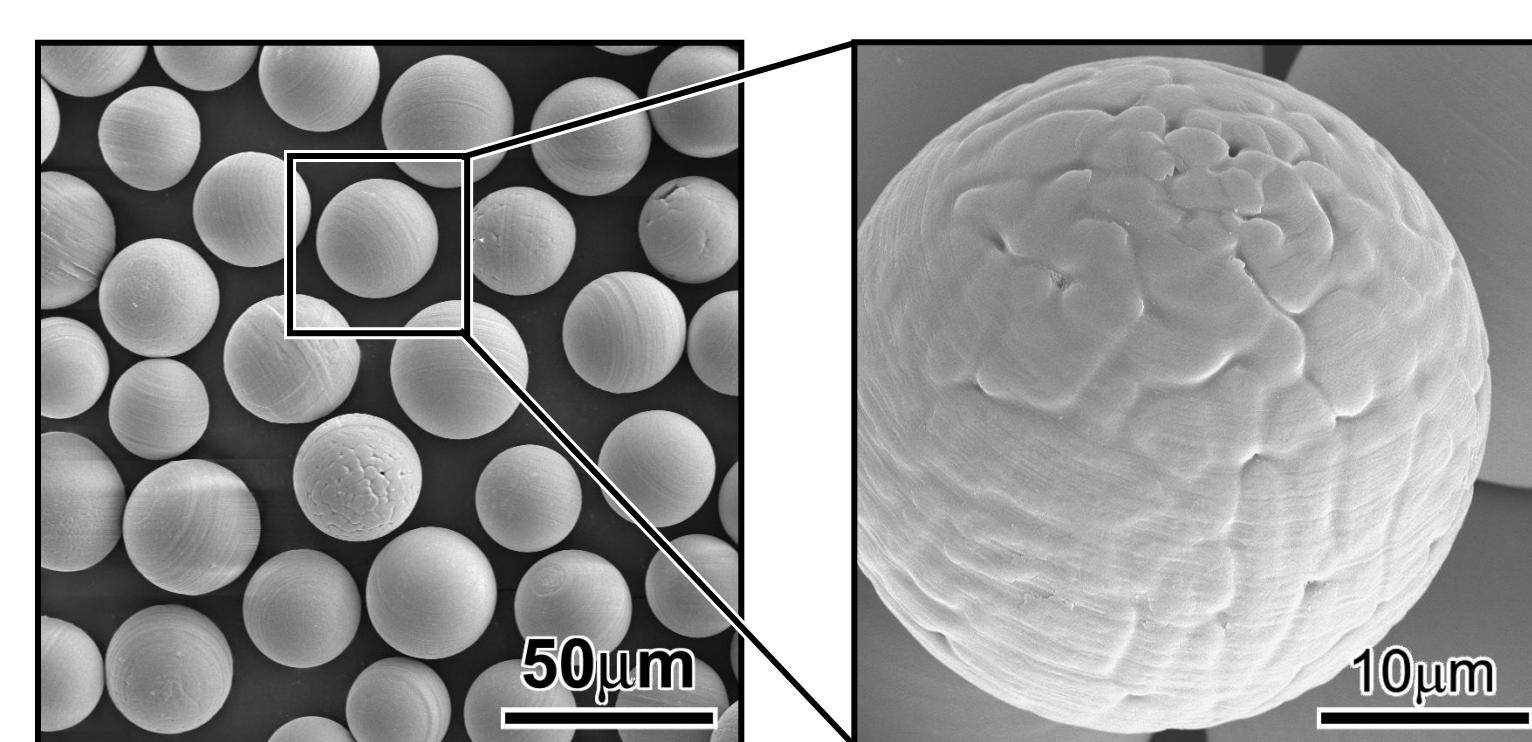
図3 \text{Y}_2\text{O}_3 微小球の走査型電子顕微鏡写真
