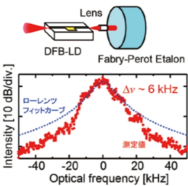
図2 光源構成とスペクトル特性
