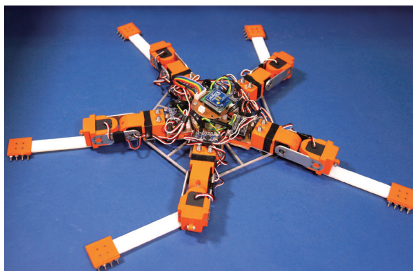
図2: 優れた耐故障性を示すクモヒトデ型ロボット
