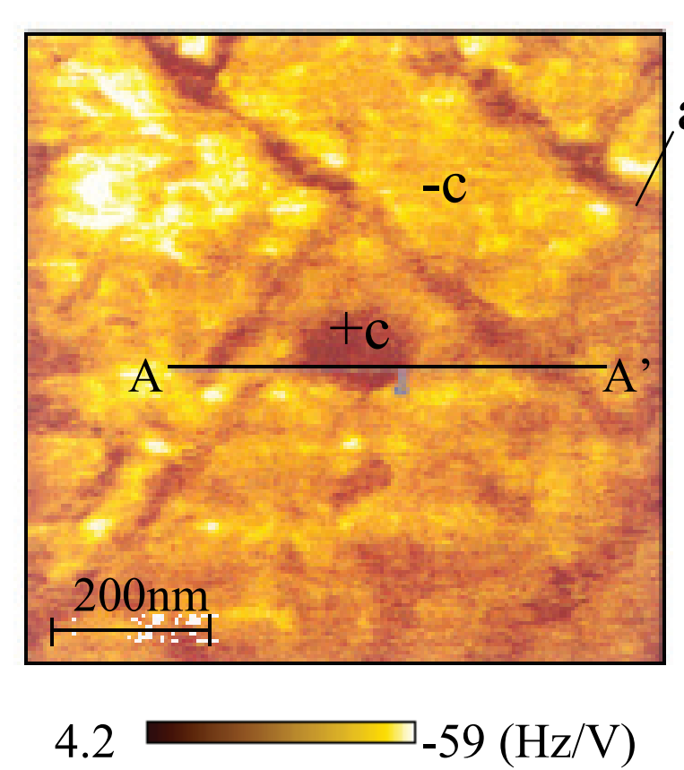
PZT薄膜のドメイン構造 (高分解能測定結果)
