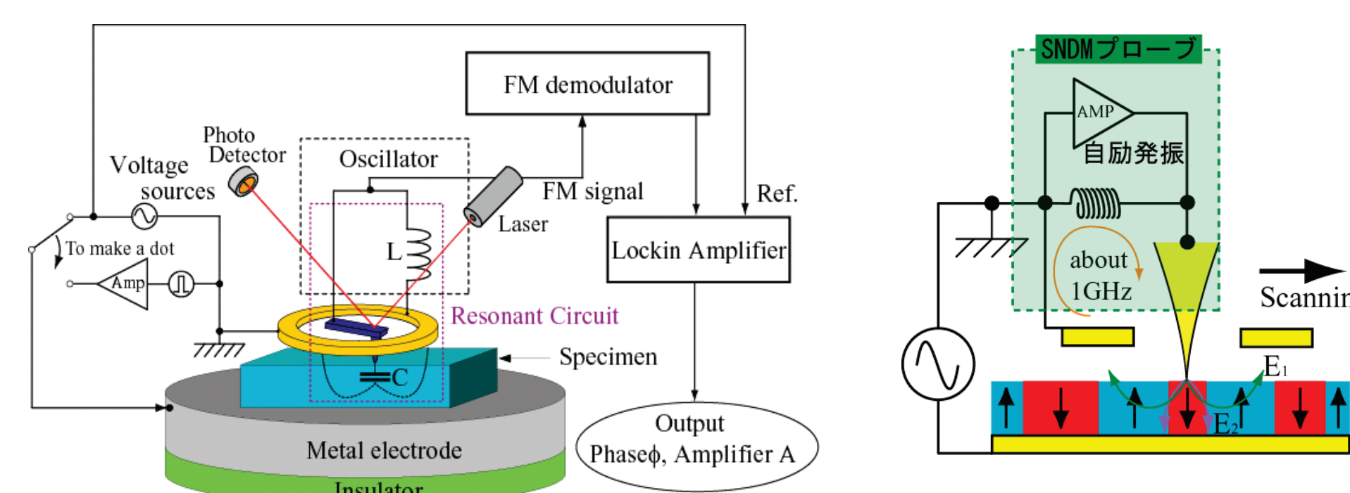
測定原理
