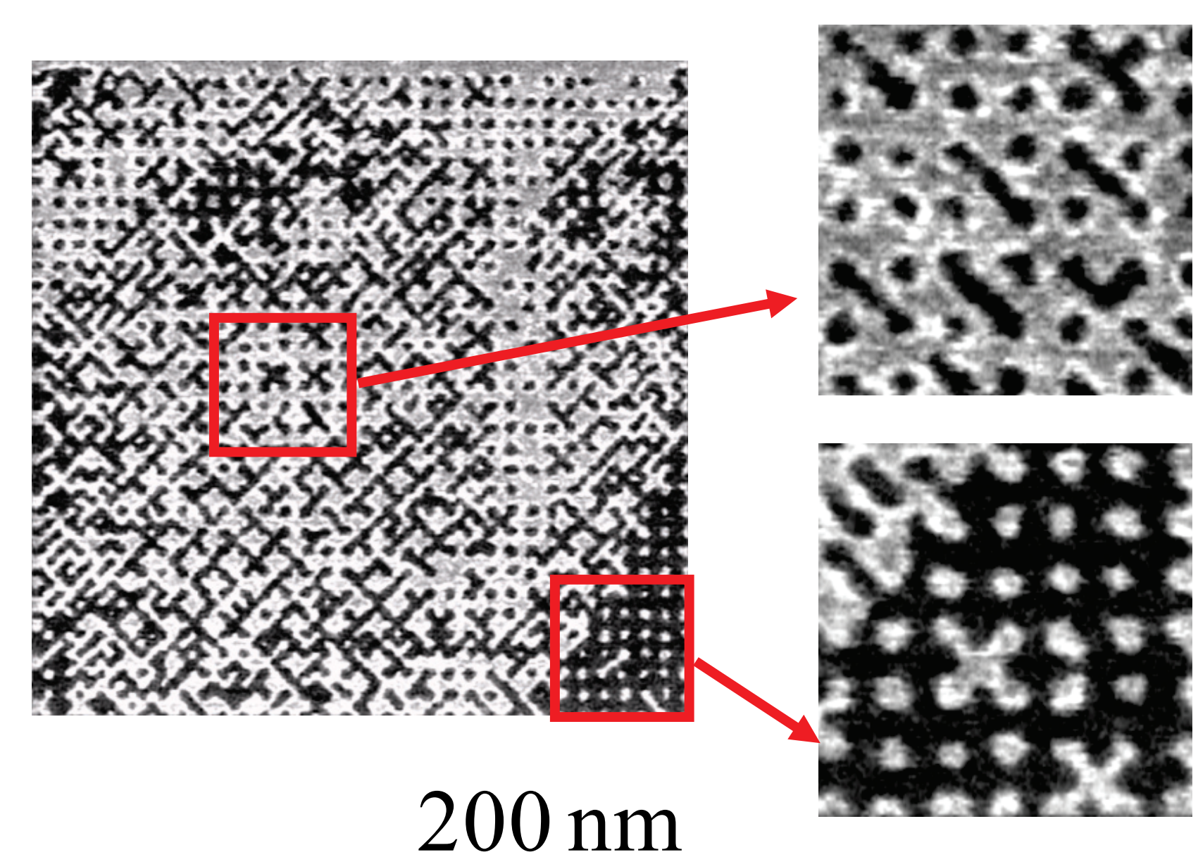
4Tbit/inch 2 での実データ記録
