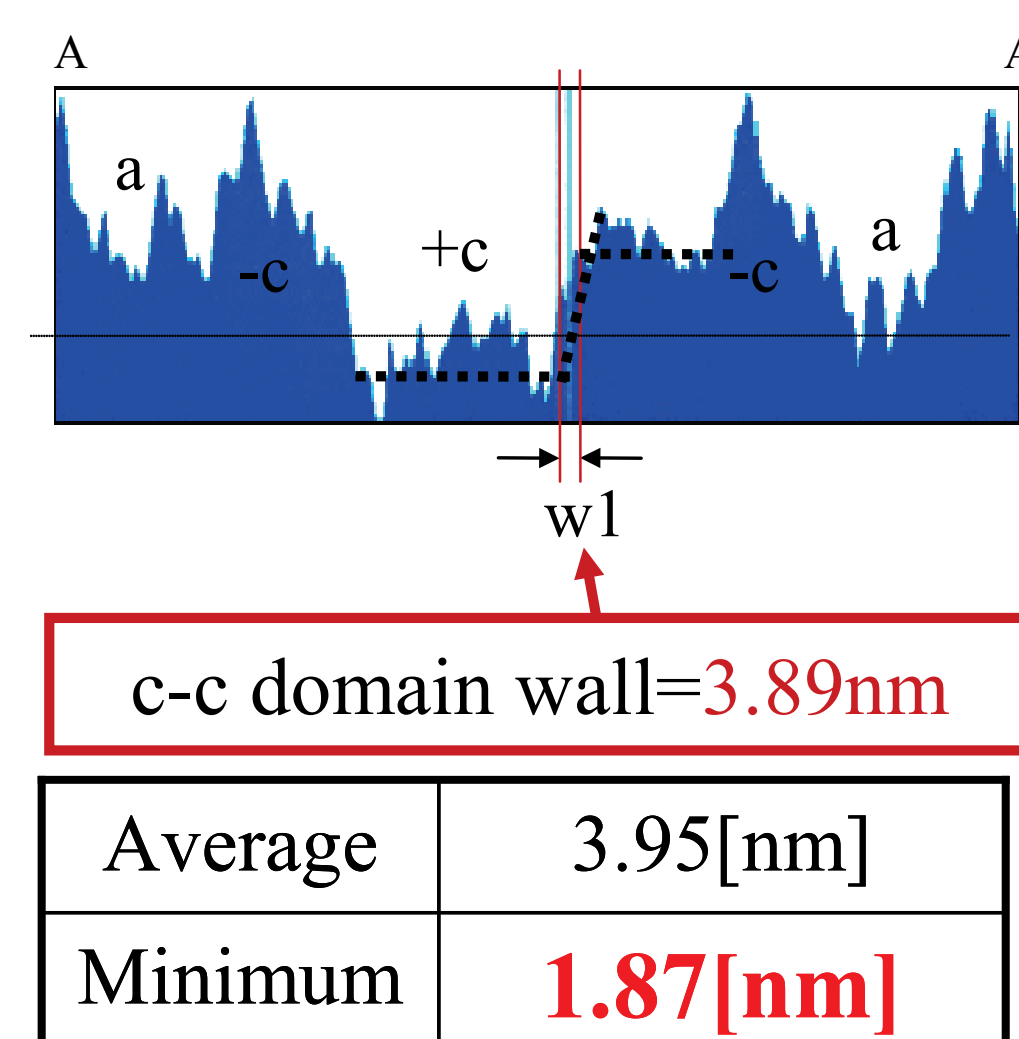
PZT薄膜のドメイン構造 (高分解能測定結果)
