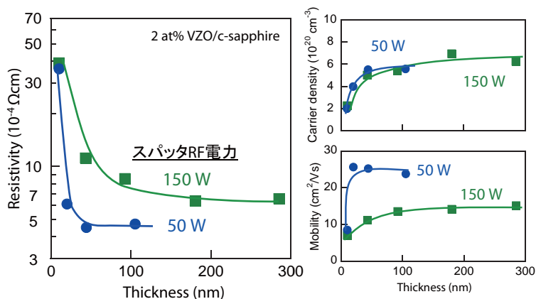
成長ドメイン制御による低抵抗VZOナノ薄膜
