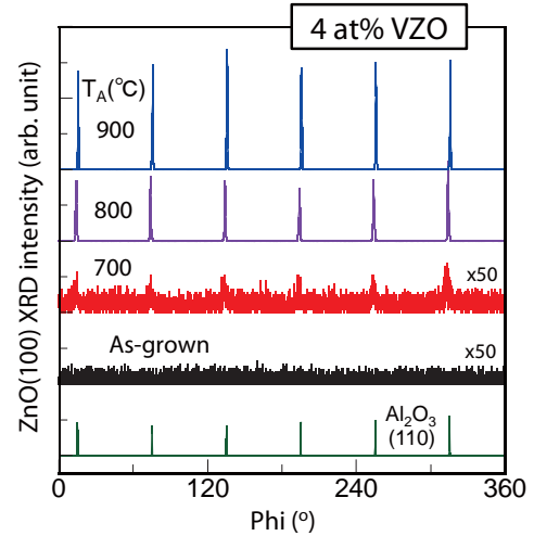
固相成長による配向化
