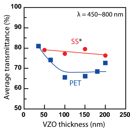
フィルム上VZOナノ薄膜の電気特性と光透過特性
