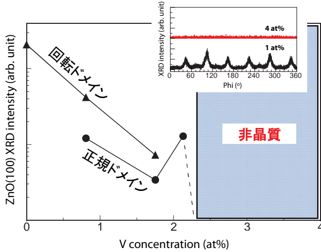
V添加による非晶質化
