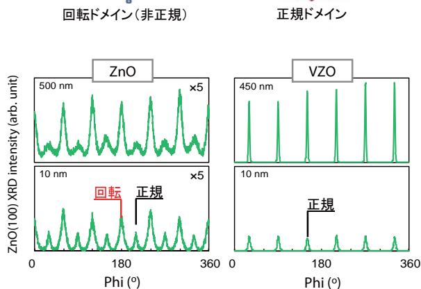
V添加による回転ドメイン成長の抑制
