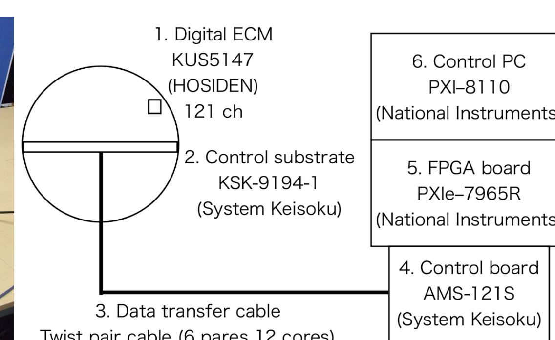
実環境の3次元音空間の収録システム
