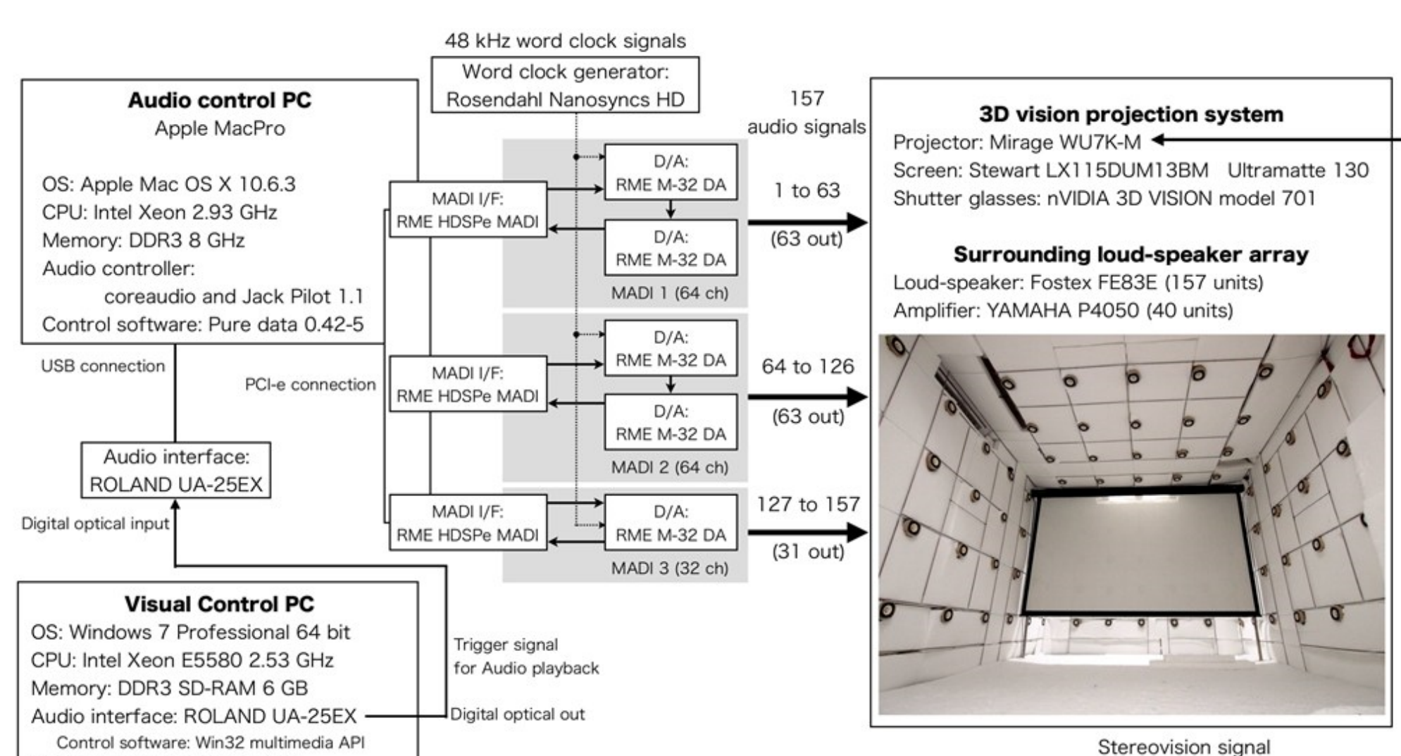
3次元視聴覚ディスプレイ
