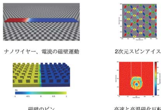
図2 マイクロ磁区シミュレーションの例 Fig.2 Examples of micromagnetic simulations
