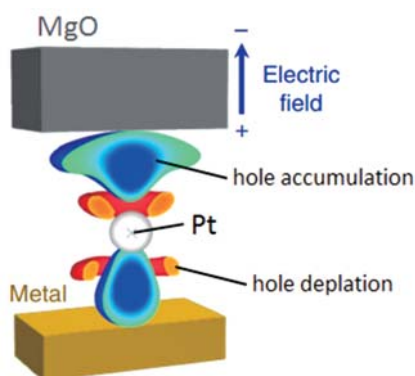
図 1: MgO/Pt/Fe 界面の Pt 原子に電圧誘起された電子分布の変化 Fig.1: Voltage-induced modulation of charge distribution of Pt atom at the MgO/Pt/Fe interface
