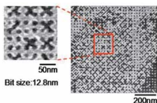
1. 微小分極反転ビットデータによる実情報記録例 (4Tbit/inch 2 ) Fig.1 Ultra-high density actual information storage using ferroelectric nano-domain manipulation (4Tbit/inch 2 )
