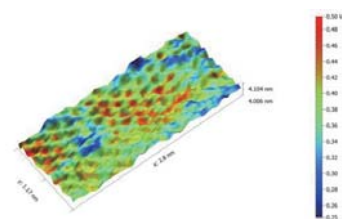
3. 超高真空非接触走査型非線形誘電率ポテンシオメトリによる SiC 上グラフェンの原子分解能観察 Fig.3 Atomic resolution imaging of graphene on SiC by ultrahigh vacuum noncontact scanning nonlinear dielectric potentiometry
