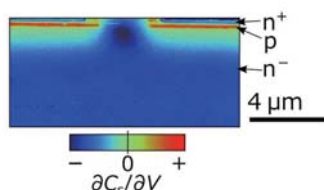
2. SiC パワー MOSFET のドーパントプロファイルの計測 Fig.2 Dopant profile measurement of SiC power MOSFET
