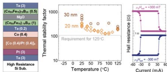
高い熱安定性を有する Co/Pt 積層構造細線における スピン軌道トルク磁化反転
