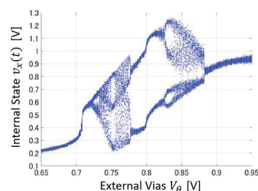
図1：(左) カオスニューラルネットワークリザーバー。(中) 3D 積層集積回路用サイクリックカオスニューラルネットワークリザーバープロトタイプチップ。(右) 測定された分岐特性 Fig.1 (Left) Chaotic neural network reservoir. (Middle) Cyclic chaotic neural network reservoir prototype chip for 3D stacked IC. (Right) Measured bifurcation diagram.
