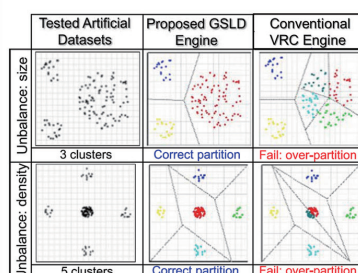
図2 提案適応型 K-means 教師無学習アーキテクチャの性能検証と比較: アンバランスなデータに対する大幅な学習精度向上と 88.9% 以上の計算コスト削減を実証
