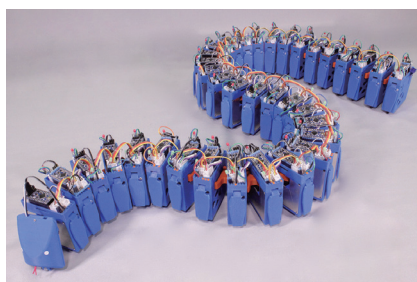
図1. 優れた環境適応性を有するヘビ型ロボットの自律分散制御
