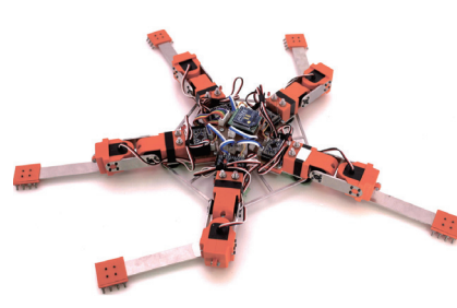
図3. 身体の一部の故障に即座に適応して推進可能なクモヒトデ型ロボット
