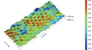
3. 超高真空非接触走査型非線形誘電率ポテンシオメトリによる SiC 上グラフェンの原子分解能観察
