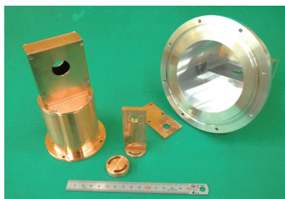
図1 クライオスタット シュラウド & 輻射シールド
