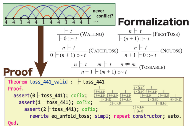
図2 定理証明支援系による「ジャグリングの数学」の形式化
