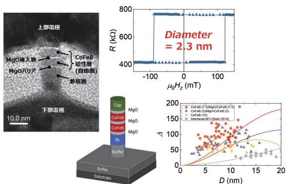
不揮発性メモリ向け世界最小・高性能磁気トンネル接合素子 The world-smallest magnetic tunnel junction for nonvolatile memory
