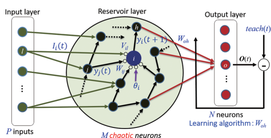
図1：(左) カオスニューラルネットワークリザーバー。(中) 3D 積層集積回路用サイクリックカオスニューラルネットワークリザーバープロトタイプチップ。(右) 測定された分岐特性 Fig.1 (Left) Chaotic neural network reservoir. (Middle) Cyclic chaotic neural network reservoir prototype chip for 3D stacked IC. (Right) Measured bifurcation diagram.
