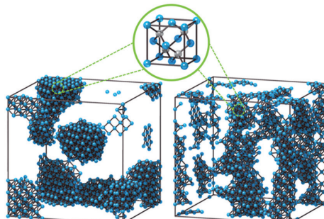
図2: スピノードル分解により形成された強磁性半導体 (In, Fe) Sb の大理石相(左)と昆布相(右)
