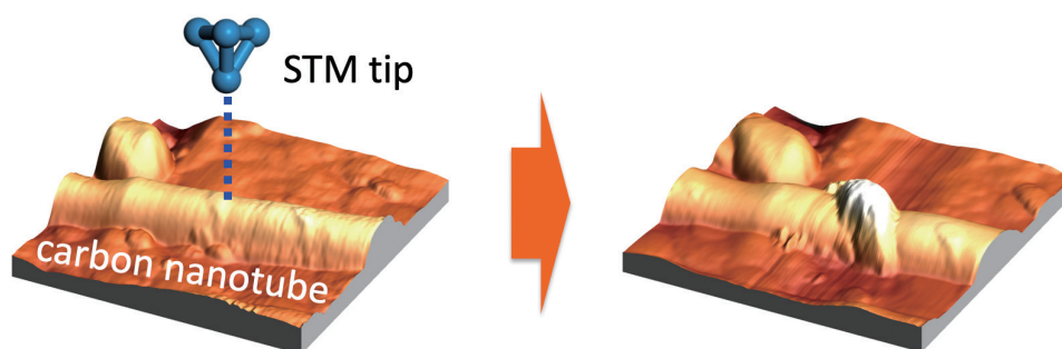
走査トンネル顕微鏡 (STM) によるカーボンナノチューブ鎖上へのナノ構造形成 Fabrication of a nanostructure on the carbon nanotube using scanning tunneling microscope (STM)
