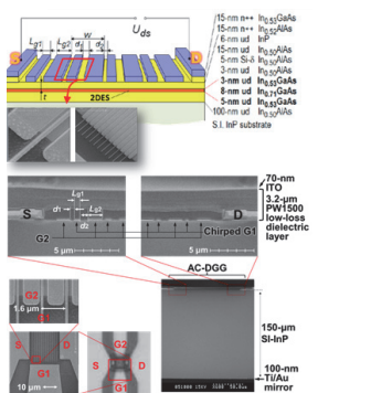
2次元プラズモン共鳴効果を利用したInP系ヘテロ接合材料による新しいテラヘルツ帯エミッタ・ディテクタ素子 (A-DGG-HEMT) の断面構造、電子顕微鏡写真 Cross-sectional view and SEM images of an InP-based asymmetric dual-grating-gate (A-DGG) HEMT.
