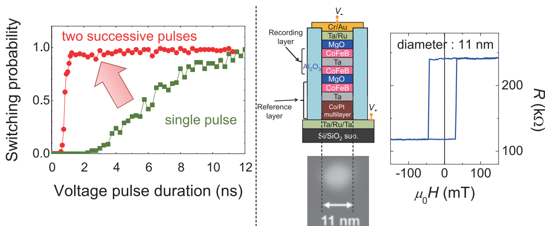
(左) 従来の単一電圧パルスを用いたメモリ操作手法（緑）と新たに開発した二段パルスを用いたメモリ操作手法（赤）に対する磁化反転確率の入力電圧継続時間（≒メモリ操作時間）依存性。（Applied Physics Letters 2014） (右) 世界最小（直径 11 nm）の MTJ の模式図と走査型電子顕微鏡像、およびその素子動作特性。
