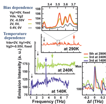
A-DGG HEMT 素子からの世界初の単色コヒーレントテラヘルツ放射の観測結果 Record-breaking world-first coherent, monochromatic THz emission from the A-DGG HEMT.
