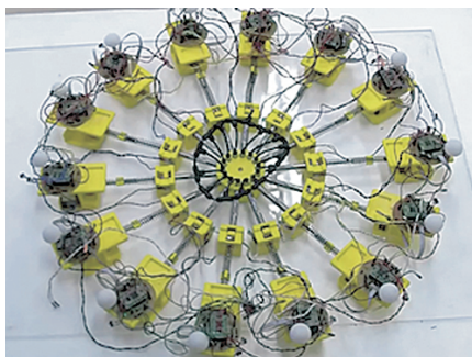
真正粘菌変形体をモチーフとして製作した完全自律分散制御で駆動するアメーバ様ロボット
