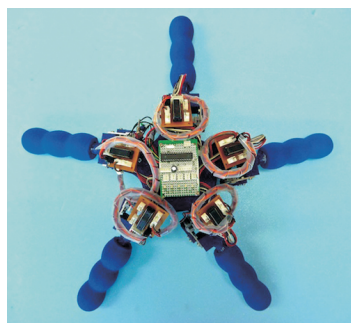
腕を自発的に役割分担して全方向移動可能なクモヒトデ型ロボット
