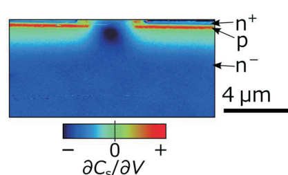
図3. SiC パワー MOSFET のドーパントプロファイルの計測
