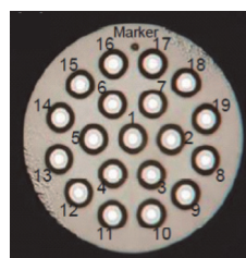
2048 QAM コヒーレント光信号 (左) および 19 コアファイバの断面写真 (右) 2048 QAM coherent optical signal (left) and cross section of 19-core fiber (right)
