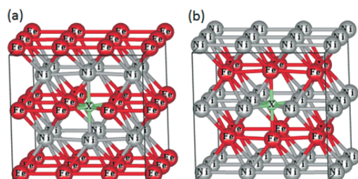
図 1: Fe (a) または Ni (b) 原子層の格子間八面体位置に軽元素原子を添加した L1_0 -FeNi 合金のスーパーセルの模式図。
