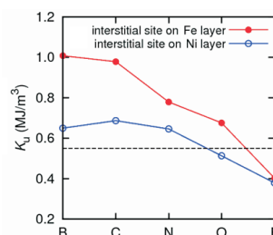
図 2: 軽元素 (B, C, N, F, O) を 2.6 at% 添加した L1_0 -FeNi 合金の一軸結晶磁気異方性エネルギー ( K_u )。破線は軽元素を添加していない L1_0 -FeNi 合金の K_u を表している。
