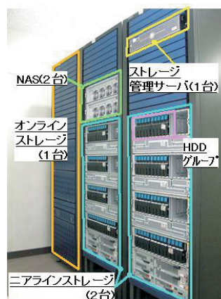
図2 多数の並列HDDにより構成される大規模ストレージシステム Fig. 2 A large-scale storage system with parallel HDD operation.
