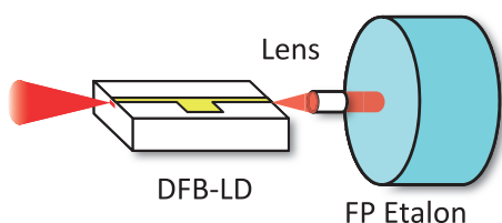
超小型狭線幅半導体レーザ光源の構成 Schematic structure of a compact narrow linewidth semiconductor laser
