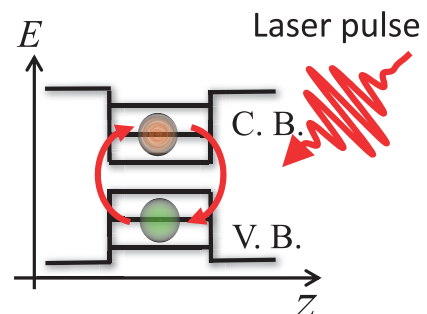
図2. 半導体量子ドット中の電子・正孔対の光学的コヒーレント制御。 Fig. 2 Coherent optical control of an electron-hole pair in a semiconductor quantum dot.
