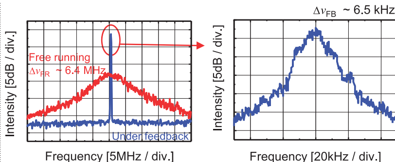
単体 DFB レーザの発振スペクトル (赤線) と帰還時の超小型狭線幅半導体レーザ光源の発振スペクトル (青線) Spectra for solitary DFB laser (red line) and for compact narrow linewidth semiconductor laser under feedback condition (blue line)
