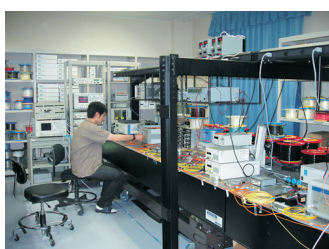
超高速光通信実験の様子
