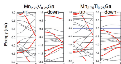
図2: D0_{22} 型 Mn_{2.75}V_{0.25}Ga (左図) および Mn_{2.75}Ti_{0.25}Ga (右図) のバンド分散。赤線は \Delta_1 バンドを表し、エネルギー(縦軸)の原点はフェルミ準位に取られている。
