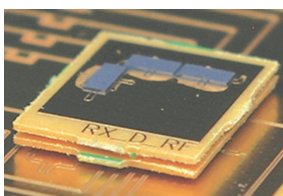
Fig. 2 ハイビジョン非圧縮伝送超小型 3D SiP ミリ波無線端末 Fig. 2 Ultra-small-size 3D SiP millimeter wave wireless terminal for uncompressed HDTV
