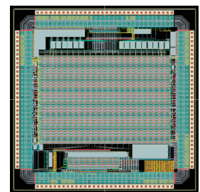
図2：(左) 従来のデジタルコンピュータが得意な組合せ最適化問題を、カオス的な迷いと直感で高速に解くカオスニューロコンピュータプロトタイプ (右) 左のプロトタイプを小型化・高速化して大規模な実用問題に対応できるようにするためのVLSIチップ Fig. 2 (Left) A chaotic neuro-computer proto-type system for quadratic assignment problems, which uses chaotic wanderings and inspirations to find solutions. (Right) A dedicated VLSI chip for a fast and practical large-scale chaotic neuro-computer system which can solve real-world problems.
