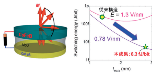
電界による磁化制御を応用した、世界最小の電力で動作するスピンメモリ素子 Spintronics device with the world's smallest switching energy with electric field control of magnetization.
