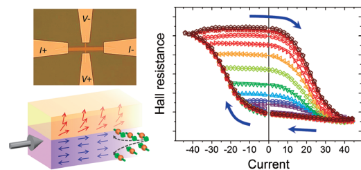
アナログ的に動作する反強磁性体を用いたスピンメモリ素子 Spintronics device with antiferromagnet that has an analogue function.
