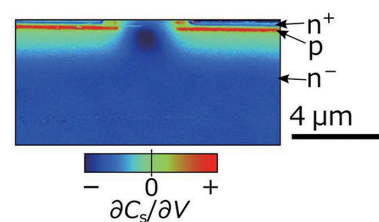
図3. SiC/パワー MOSFETのドーパントプロファイルの計測
