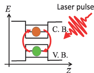
図 2. 半導体量子ドット中の電子・正孔対の光学的コヒーレント制御。
