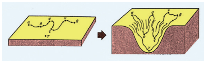
等式推論による証明 → 書き換えシステムによる計算 Proof by Equational Reasoning → Computation by Rewriting Systems
