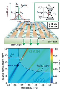
グラフェン・金属マイクロリボンアレイの表面プラズモンポラリトン励起による巨大テラヘルツ利得と超放射現象の発見 Superradiant THz lasing with giant gain in population-inverted graphene-metal ribbon arrays.
