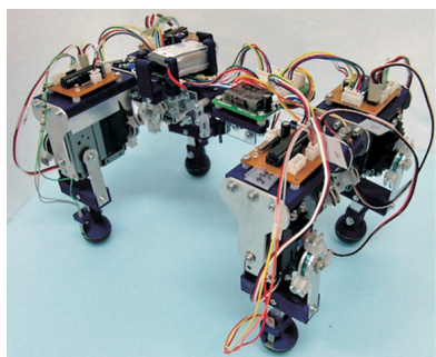
図4. 環境や身体変化に応じて自己組織的に歩行変化が変化する四脚ロボット Fig4. Quadruped robot driven by a fully decentralized control
