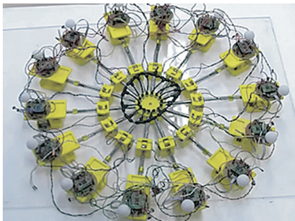
図2. 真正粘菌変形体をモチーフとして製作した完全自律分散制御で駆動するアメーバ様ロボット Fig2. Soft-bodied amoeboid robot driven by a fully decentralized control scheme extracted from true slime mold.
