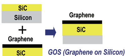
図1. 世界初のグラフェン・オン・シリコン技術 Fig1. The world-first graphene-on-silicon technology
