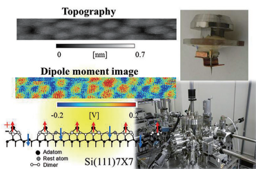
図1. 超高真空非接触走査型非線形誘電率顕微鏡によるSi(111) 7X7構造の凹凸像と双極子モーメント像
