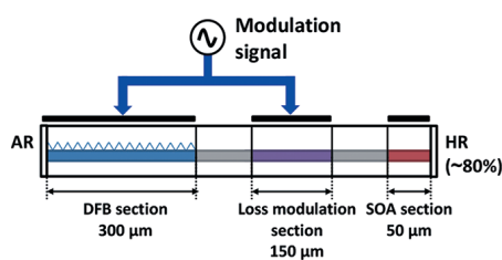
ハイブリッド変調型高速直接変調半導体レーザの構成 Schematic structure of a hybrid modulation semiconductor laser with Low-temperature STM
