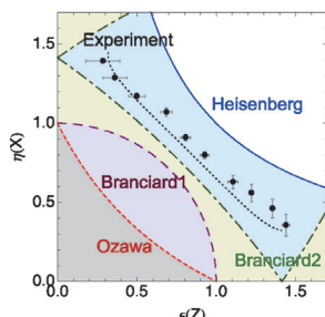
図 1. 光子の偏光測定における誤差と擾乱の不確定性関係の計測結果 (黒丸) と理論不等式の下限値 (曲線)。計測結果はハイゼンベルクの不等式 (青線) を破り、小澤 (赤) およびブランシールド (紫、緑) の不等式を満たす領域にある。
