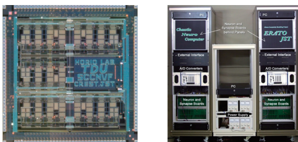
図1：(左) カオスニューロチップ (右) 1万個のニューロンを1億個のシナプスで結合可能な大規模汎用カオスニューロコンピュータハードウェアシステム
