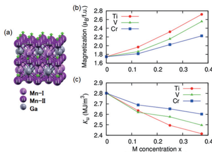
図1: (a) D0_{22} 型 Mn_3Ga の結晶構造の模式図。 Mn_{3-x}M_xGa ( M = Ti, V, Cr )の磁化(b)と一軸磁気異方性エネルギー( K_u ) (c)のM濃度依存性。
