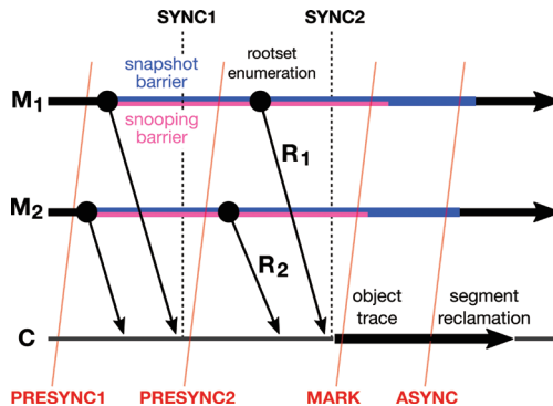
オブジェクトをコピーしない高速並行GCアルゴリズム Highly efficient fully concurrent non-moving GC algorithm
