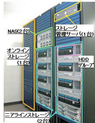
図2 多数の並列HDDにより構成される大規模ストレージシステム Fig. 2 A large-scale storage system with parallel HDD operation.
