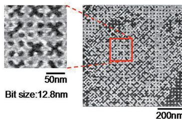
図2. 微小分極反転ビットデータによる実情報記録例(4 Tbit/inch 2 )
