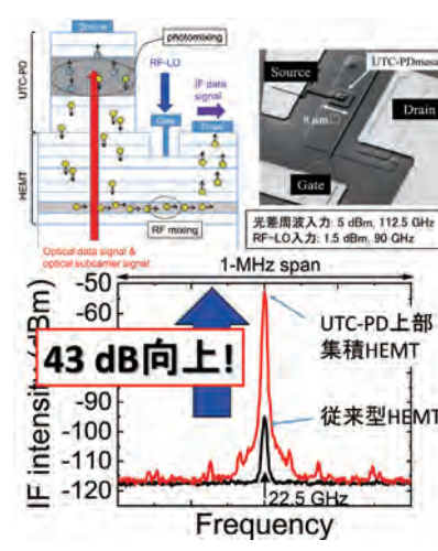
UTC-PD 上部集積 HEMT 光電子融合ミキサ素子の模式図、電子顕微鏡写真、ミキシング出力の測定結果
