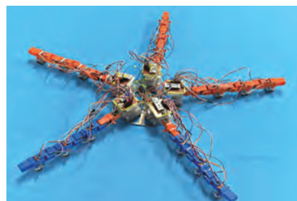
図 3. 身体の一部の故障に即座に適応して推進可能なクモヒトデ型ロボット Fig.3 Ophiuroid robot that can immediately adapt to physical damage.
