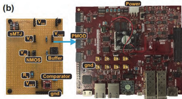
確率動作スピン素子とプログラマブル半導体回路からなる確率論的コンピューター Probabilistic computer with stochastic spintronic device and programmable CMOS circuit
