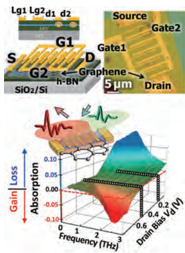
二重回折格子ゲート型グラフェンディラックプラズモントランジスタにより理論限界を4倍以上超越する巨大利得によるテラヘルツ電磁波の増幅に成功
