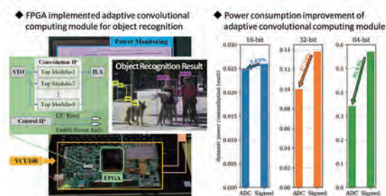
図2 8bit/16bit/32bit/64bit 混在の固定小数点処理する提案不揮発FCNN 物体検出認識プロセスにおいて、新しい適応型畳み込み演算回路を提案してFPGA実装し、消費電力優位性を確認した
