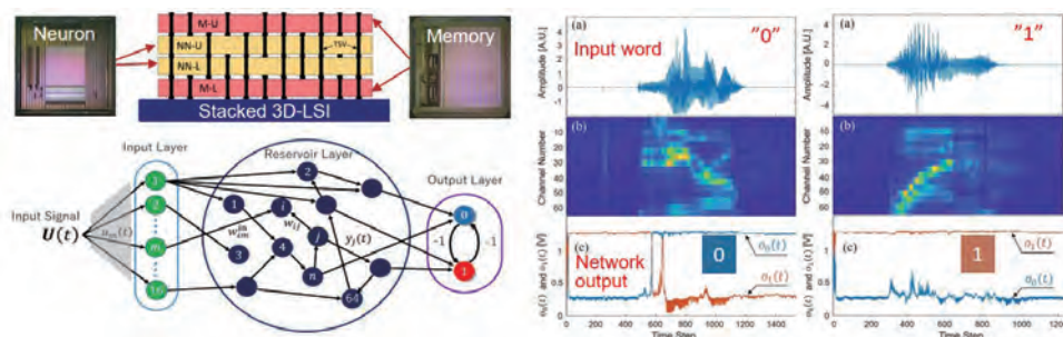
(左上) 3次元カオスニューラルネットワーク LSI。(左下) 離散単語認識実験に用いたネットワーク回路。(右) 認識実験結果。
