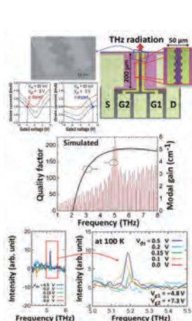
電流注入型グラフエントランジスタレーザ素子 (DFB-DG-GFET) の電子顕微鏡写真、利得係数 & Q 値解析結果、単一モードテラヘルツレーザ発振の観測結果 current-injection graphene transistor laser (DFB-DG-GFET). SEM images, measured ambipolar property, simulated modal gain and Q factor, and world-first measured single-mode THz lasing spectra.
