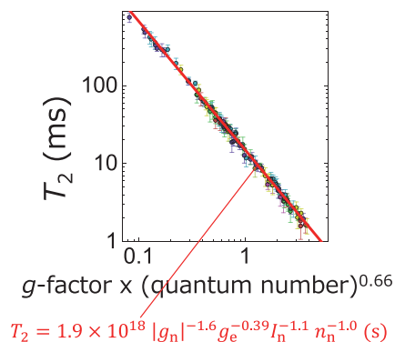
色中心スピン量子ビットのコヒーレンス時間 T_2 のスケーリング則 Scaling law of coherence time T_2 of solid-state spin qubit
