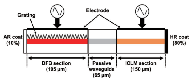
混合変調半導体レーザ
