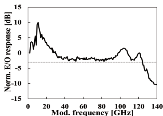
小信号応答特性 (実験値)
