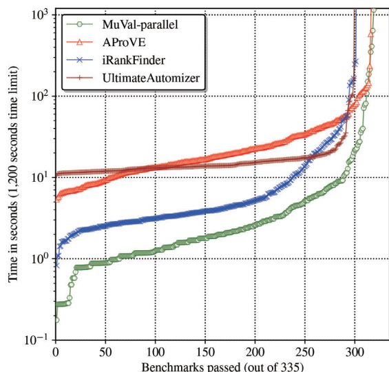
図1 開発した検証ツール MuVal の性能評価
