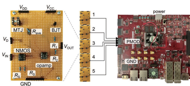
製造容易性に優れたスピントロニクス確率論的コンピュータの原理検証システム Demonstration system of manufacture-friendly spintronics probabilistic computer
