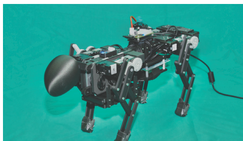
図 1. 動物のしなやかな身体構造を模倣した四脚ロボット Fig.1 Quadruped robot mimicking animal's flexible body structure
