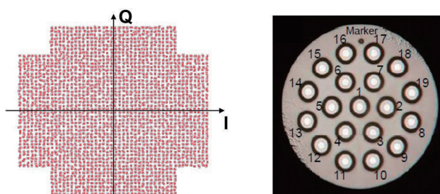
2048 QAM コヒーレント光信号 (左) および 19 コアファイバの断面写真 (右)
