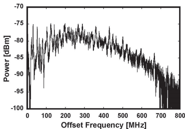
図2 マルチコアファイバ中の GAWBS 雑音スペクトル Fig.2 GAWBS noise spectrum in multi-core fiber
