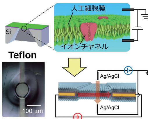
図3 人工細胞膜を用いたナノ・バイオハイブリッドシステム Fig.3 Nano-bio hybrid system based on artificial cell membranes
