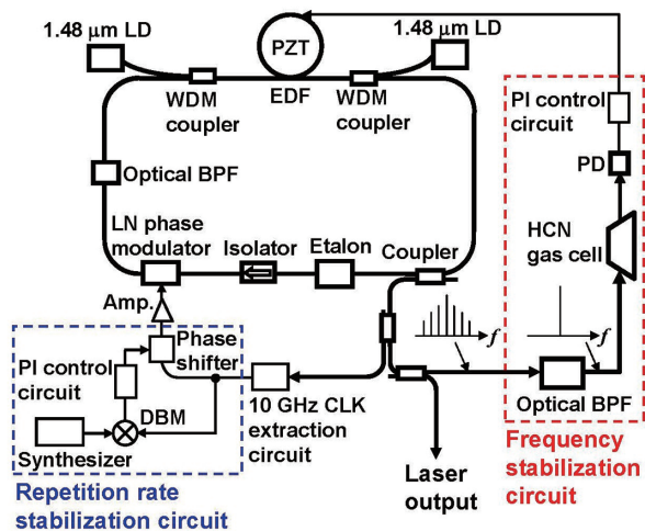
図1 1.55 \mu\text{m} 周波数安定化パルスレーザ Fig.1 1.55 \mu\text{m} frequency stabilized pulse laser
