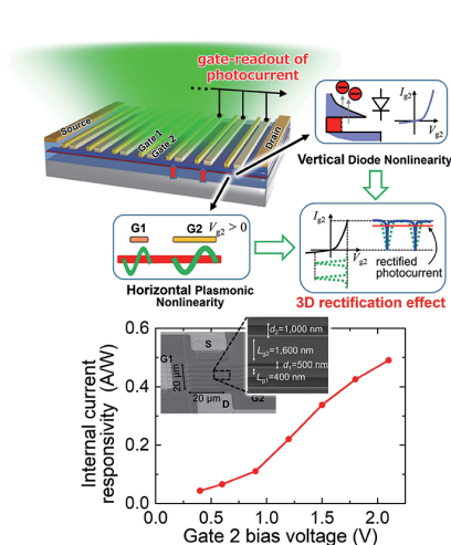
InGaAs チャンネル HEMT をベースとしたテラヘルツ・プラズモニクディテクタおよび動作原理の模式図、電子顕微鏡写真、検出感度の測定結果
