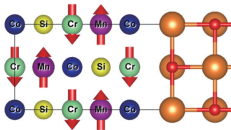
図2: 第一原理計算により高い界面磁気剛性率を有すると予測されたCoCrMnSi/MgO接合の結晶構造と磁気構造の模式図
